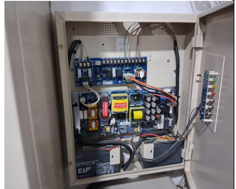
중계기 전원반(내부 모습)
