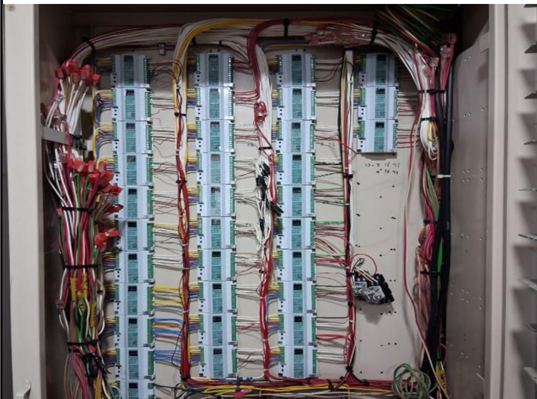
중계기 집합함 내부(중계기 전원공급안됨)
